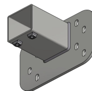
Vægbeslag fod inkl. væg/spær montage 691209-57
