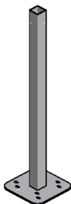
Stolpe 90 x 90 x 4 mm med fodplade - midt længde 300 cm 691299
