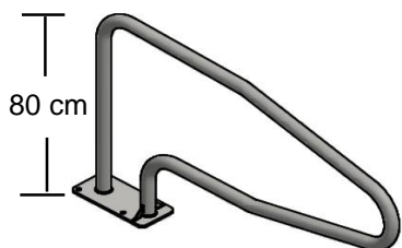
1 1/2" ungdyr op til 200 kg 690580 L=135 cm
