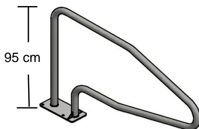
1 1/2" ungdyr 200-300 kg 690581 L=145 cm
